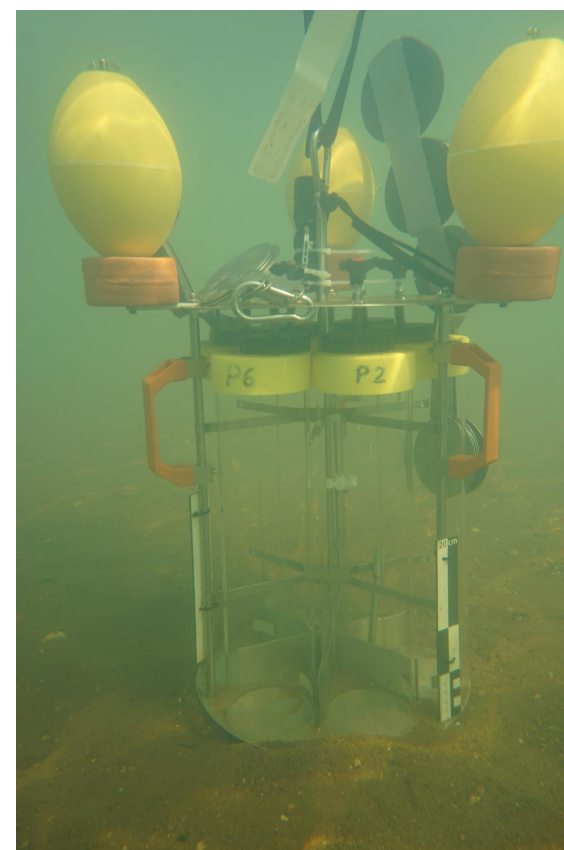
Konstruktionsmodell und Umsetzung des UWTT mit Schwimmkörpern
